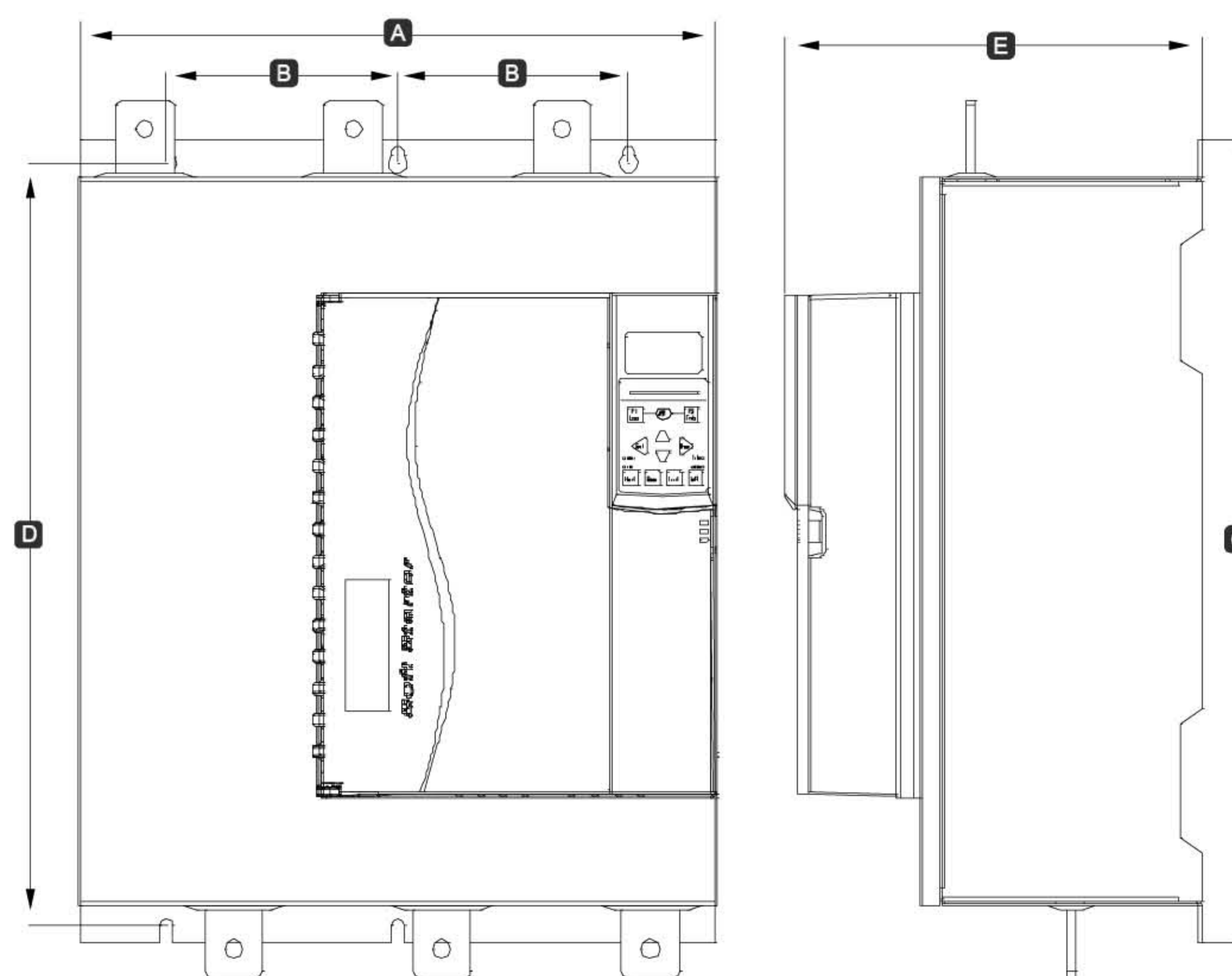
920A ~ 1600A
